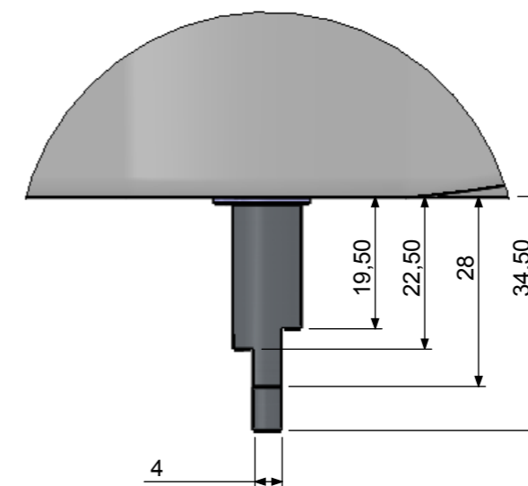
DÉTAIL A ECHELLE 1 : 1
