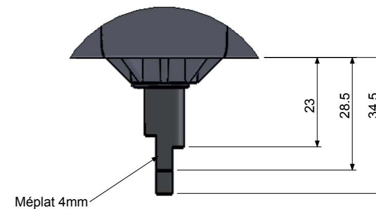
DÉTAIL A ECHELLE 1 : 1
