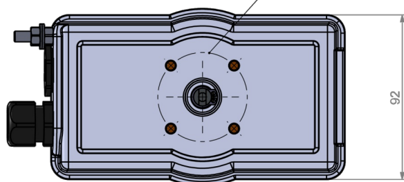
4xM6 sur Ø50(F05)
