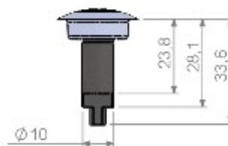
DÉTAIL A
